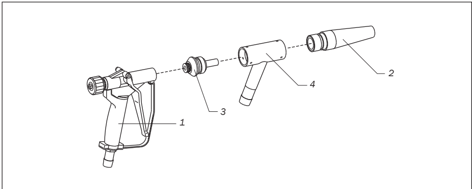
Abb. 9.1.1 Strahlpistole – Aufbau
